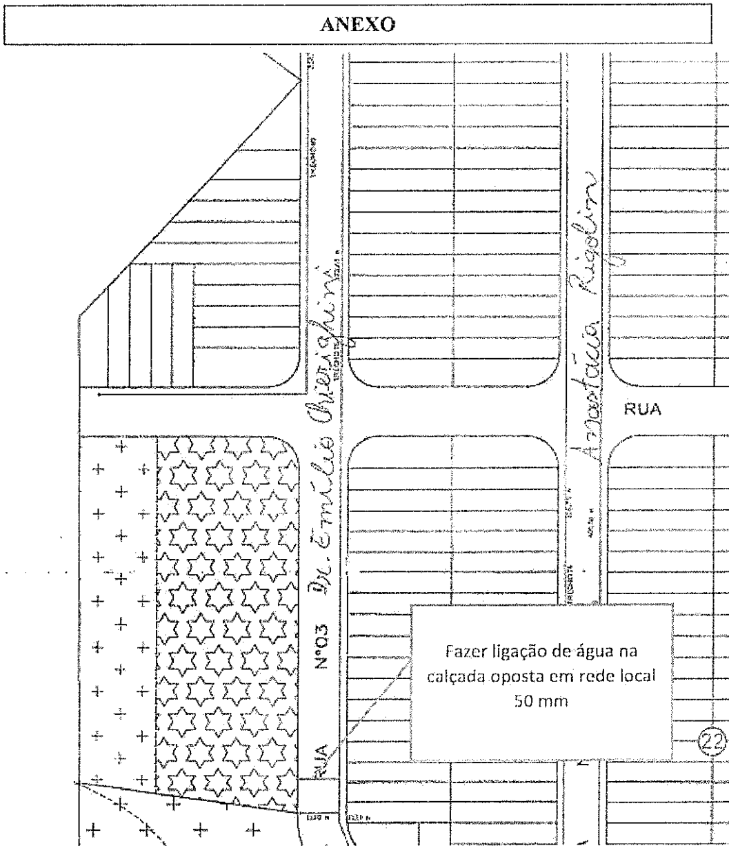
Figura 1 - Ligação de água
