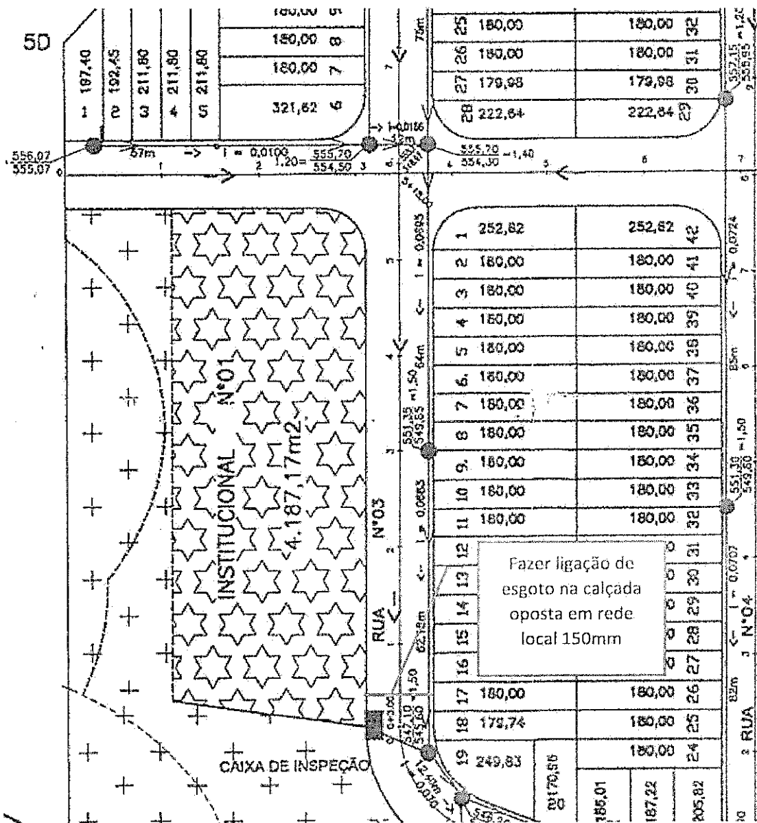
Figura 2 - Ligação de Esgoto
