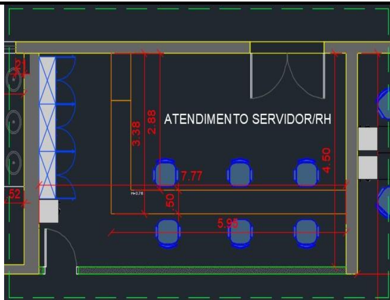
Projeto balcão para a ÁREA DE ATENDIMENTO SERVIDOR/RH
