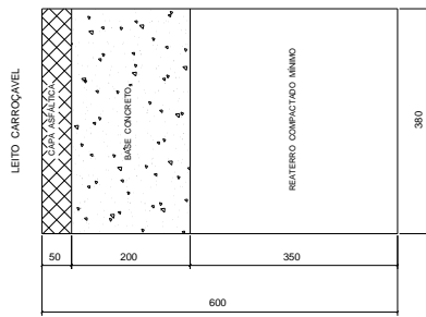
REPOSIÇÃO ASFÁLTICA - VALA DE TIPO A.
